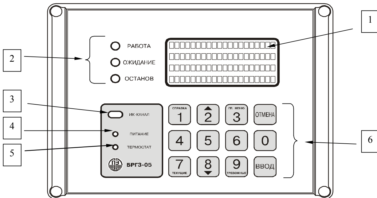
Рисунок 1 Лицевая панель блока управления
