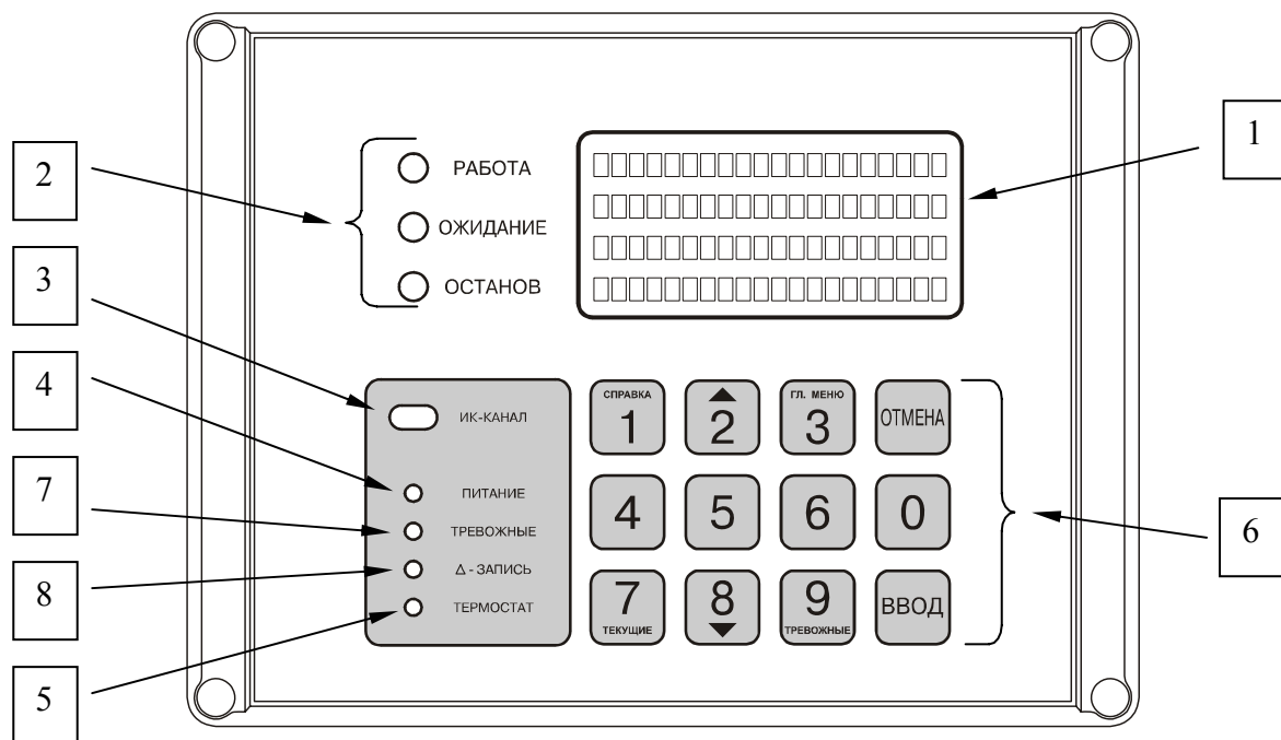
Рисунок 1 Лицевая панель блока управления
